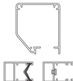
ROLO dveřní magnet box extrudovaný 48 × 42 mm
