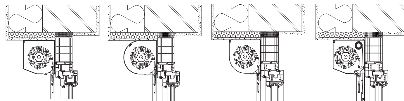
Obr. 1 - Roleta s boxem 20°
